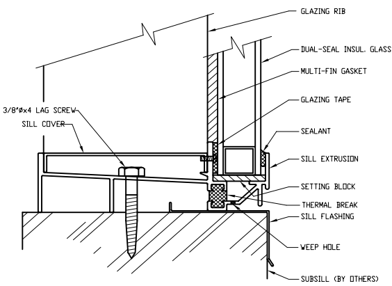
9 MAIN SILL SCALE: NONE
