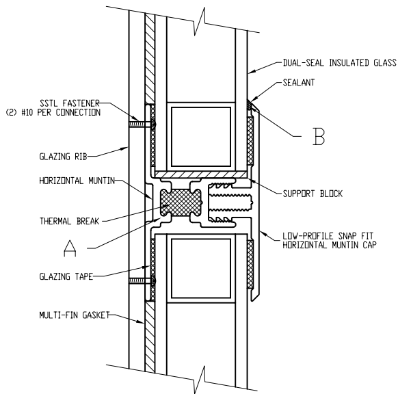
1 HORIZONTAL MUNTIN SCALE: NONE
