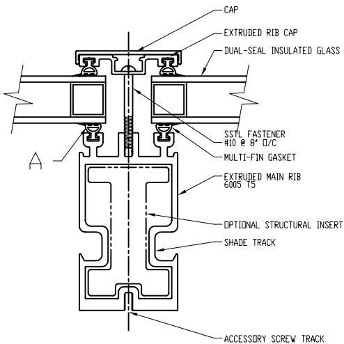
4 MAIN RIB SCALE: NONE
